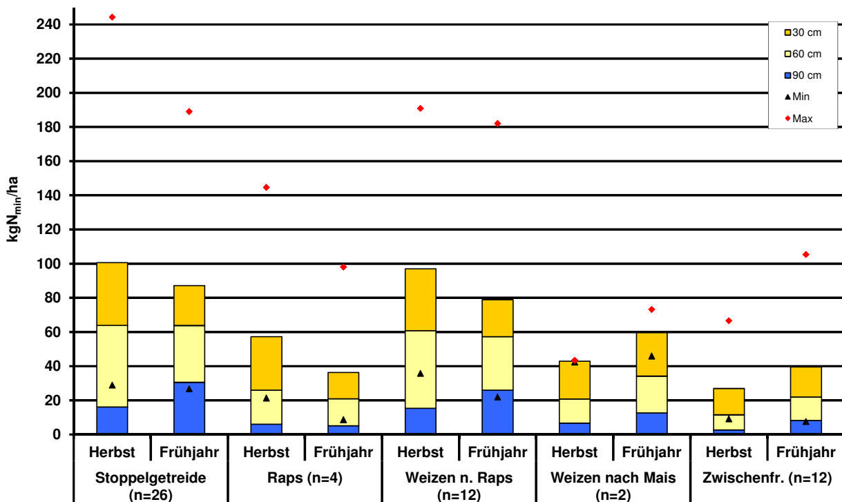
Abbildung 1: Vergleich der N min -Werte vom Herbst 2016 mit den aktuellen Werten 2017.
